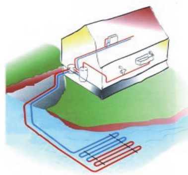
Vesistöt lämmönlähteenä
