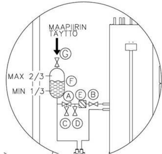
Paineistamaton maapiiri
