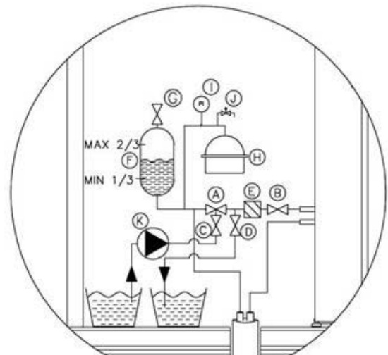
Paineistettu maapiiri
