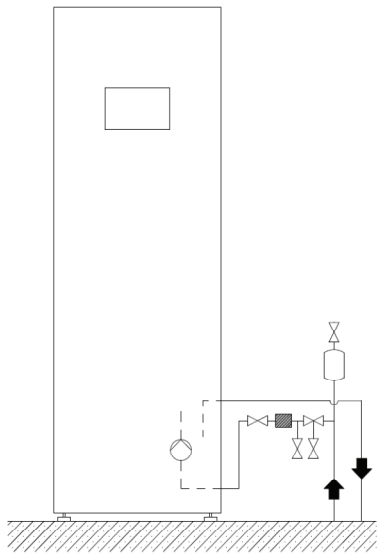
Kytkentä oikealta/takaa
