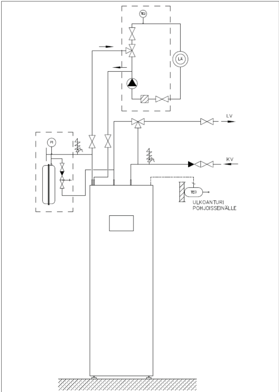
Yllä olevassa kuvassa on esitetty maalämpöpumpun kytkentä ilman käyttöveden kiertoa.
