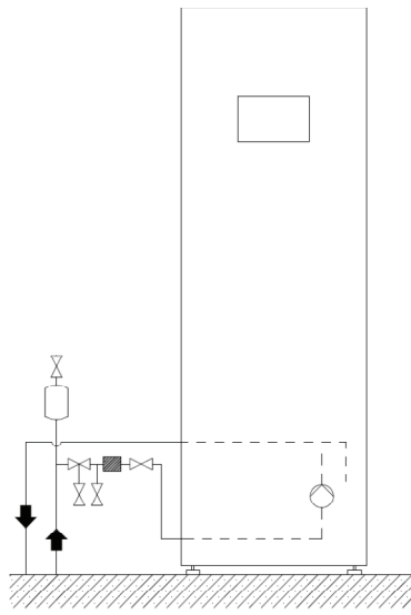
Kytkentä vasemmalta/takaa
