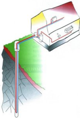
Porakaivo lämmönlähteenä
