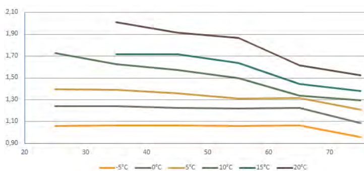
Latauspiirin virtaama dT8 [l/s]
