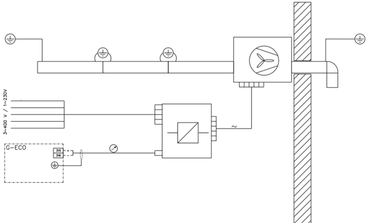
Kuva 7.5 Poistoilmamurinin kytkentäkaavio
