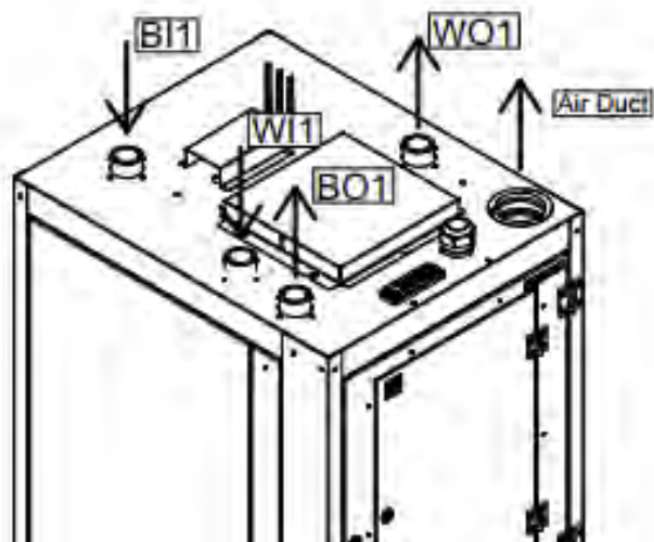
Kuva 6.1 Lämpöpumpun putkilähdöt
