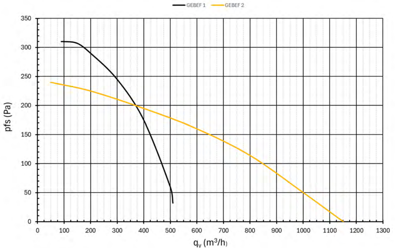
Kuvaaja 5.1 Poistoilmaimureiden suoritusarvokuvaajat
