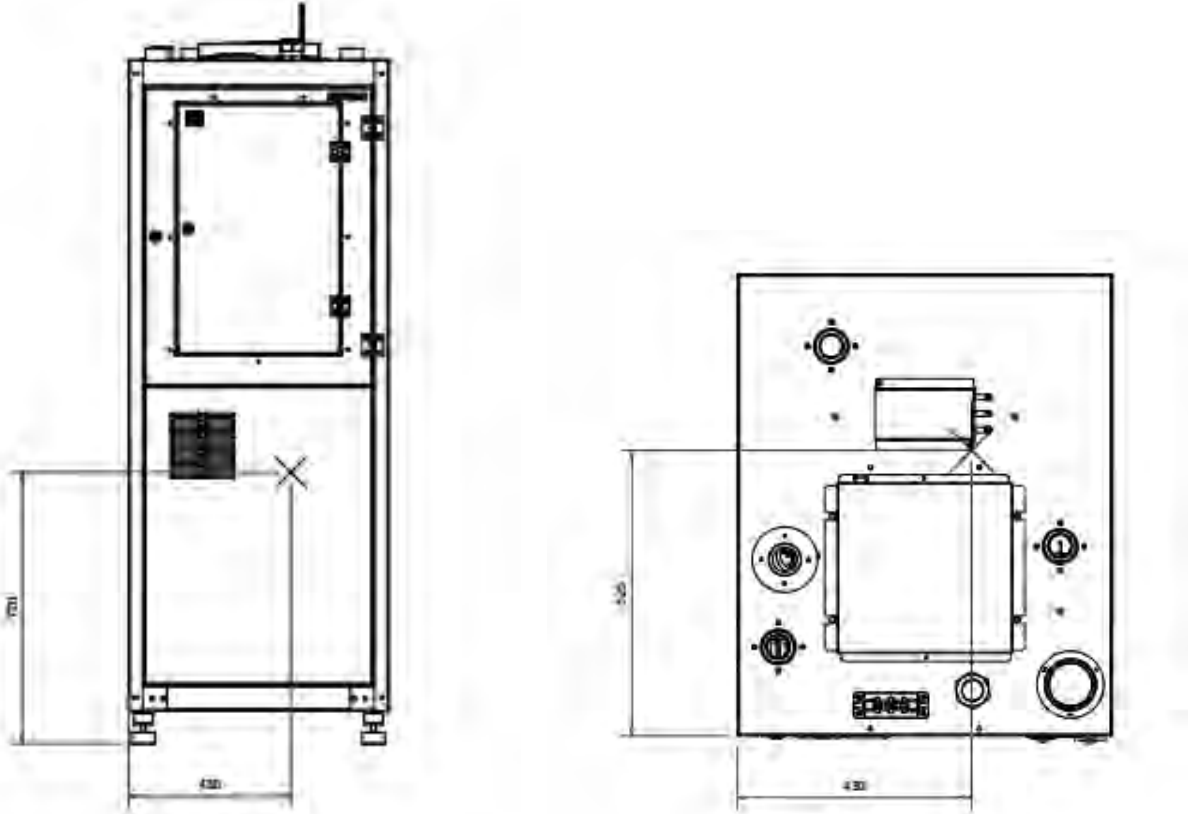
Kuva 5.1 Lämpöpumpun painopiste
