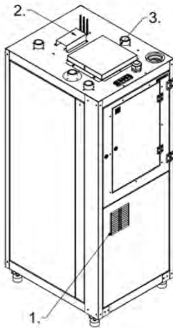
Kuva 3.3 Laitteen ulkopuoliset Komponentit ja ilmakeinavat
