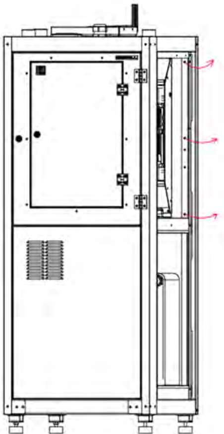
Kuva 5.17 Takaoven poistaminen
