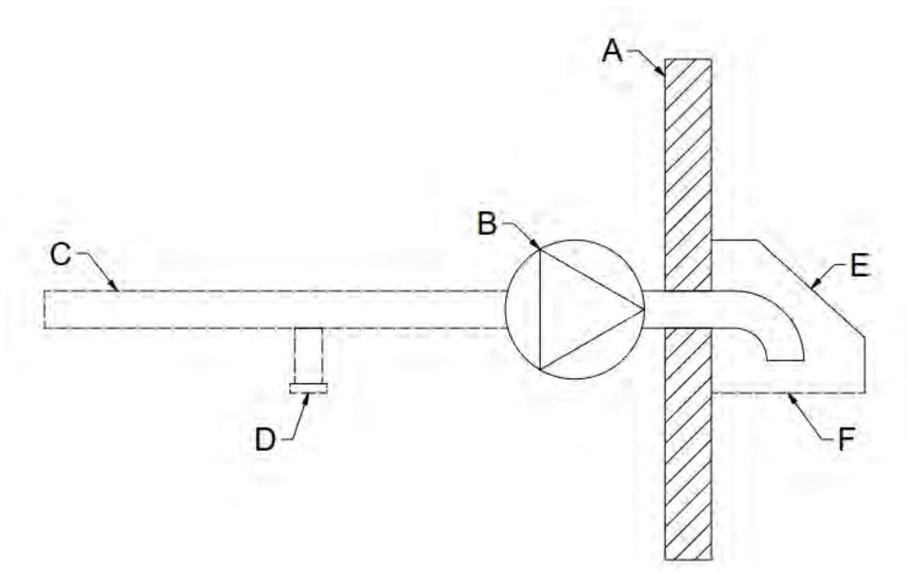
Kuva 5.11 Ilmanvaihdon ulospuhallus
