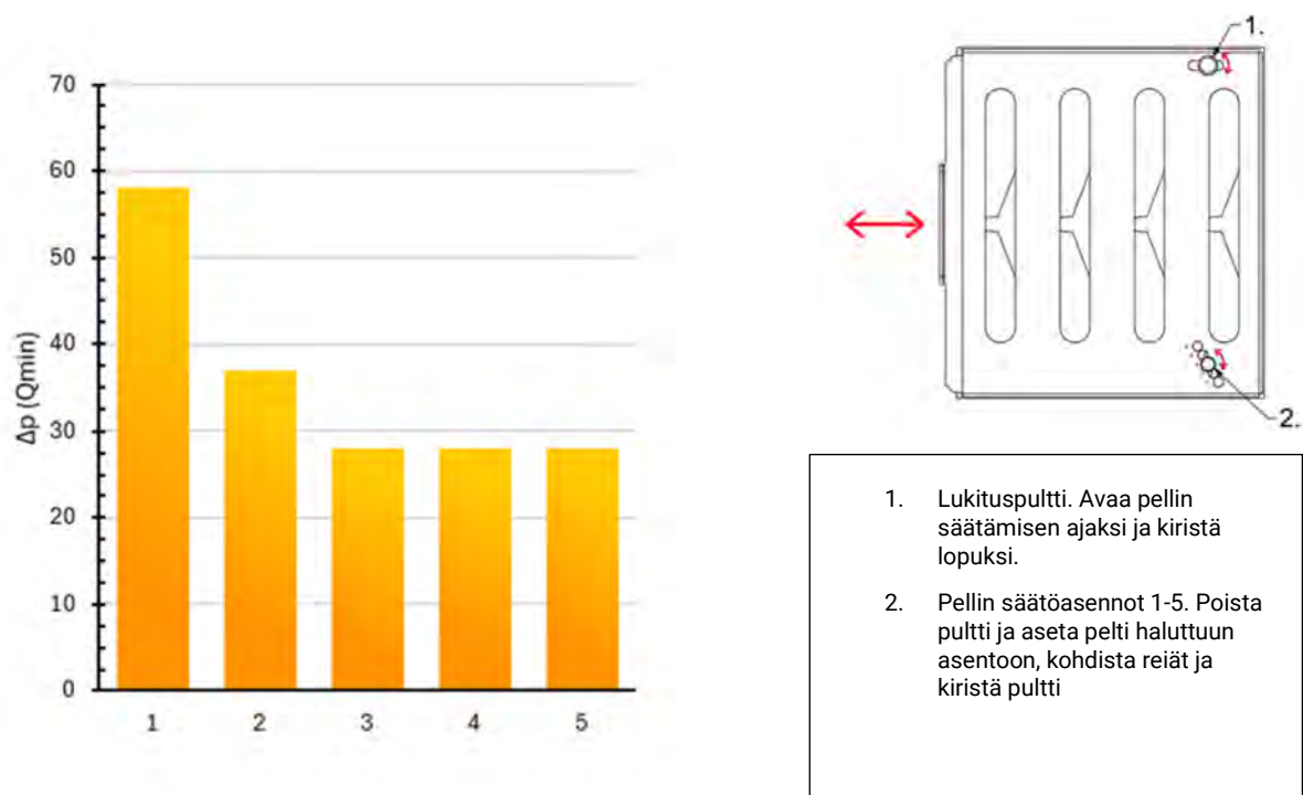
Kuvaaja 5.2 Laitteen sisäinen painehäviö ilmanvaihdolle Q_{min} virtaamalla (säätöpellin asennot 1–5)
