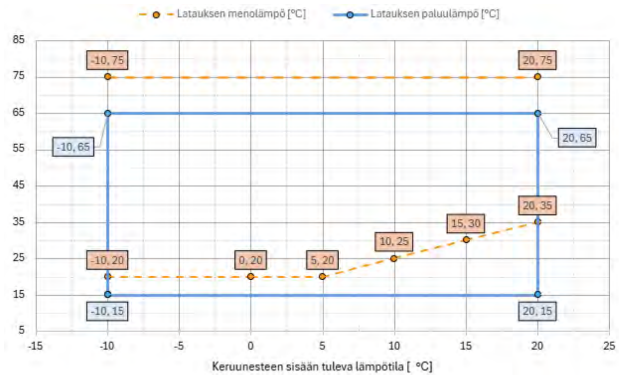
Kuva 12.1 Käyttöalue
