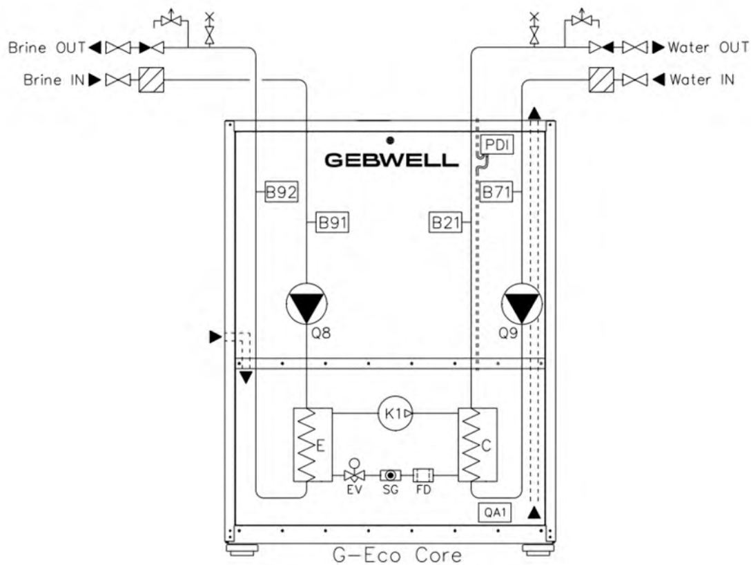
Kuva 6.2 Putkikytkentöjen mallikaavio
