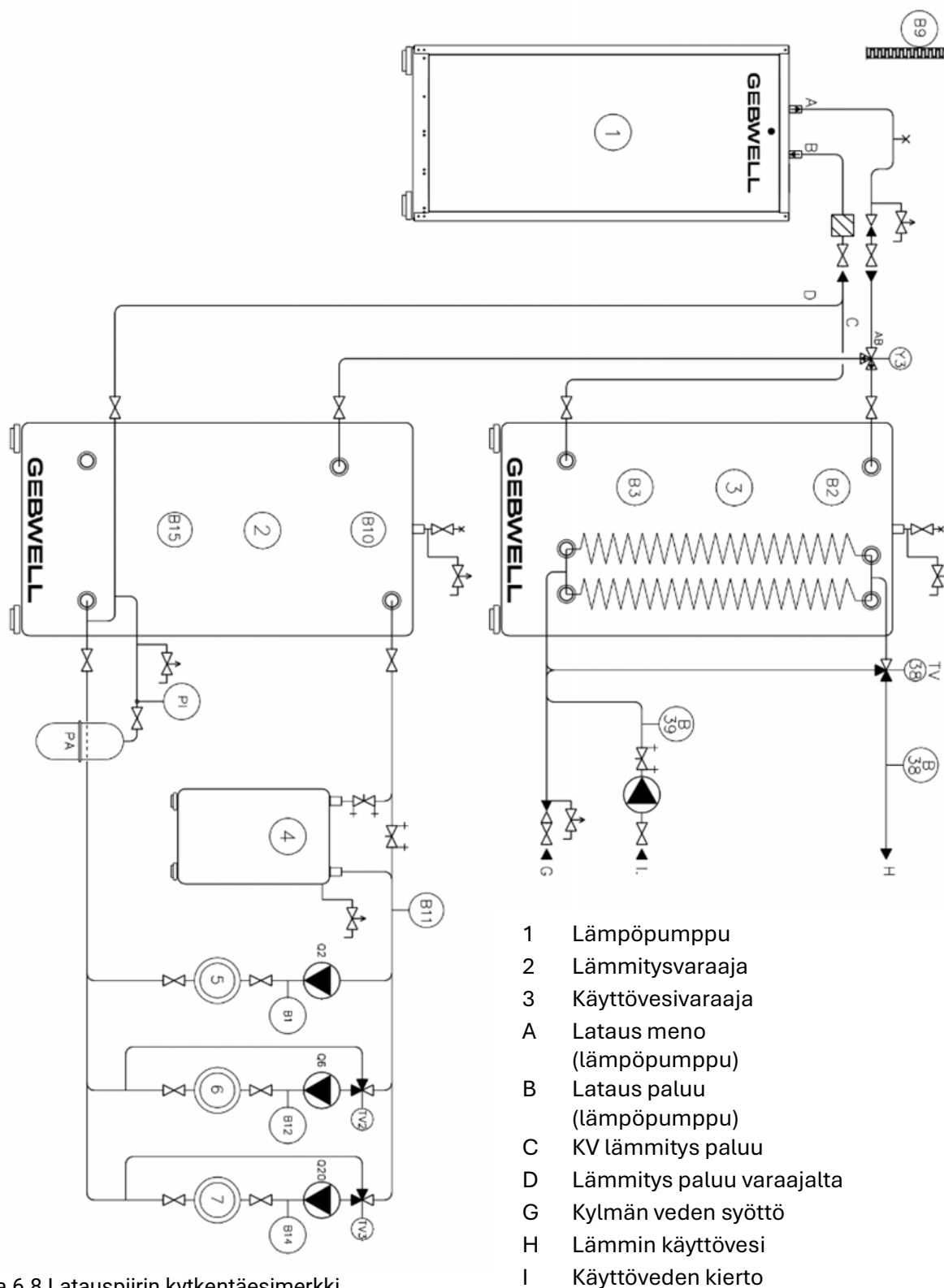
Kuva 6.8 Latauspiirin kytkentäesimerkki
