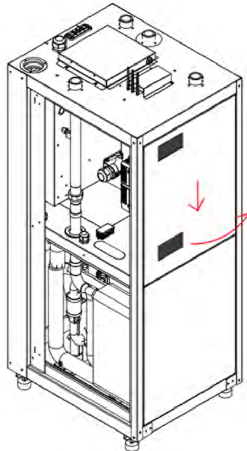
Kuva 5.18 Takaoven poistaminen
