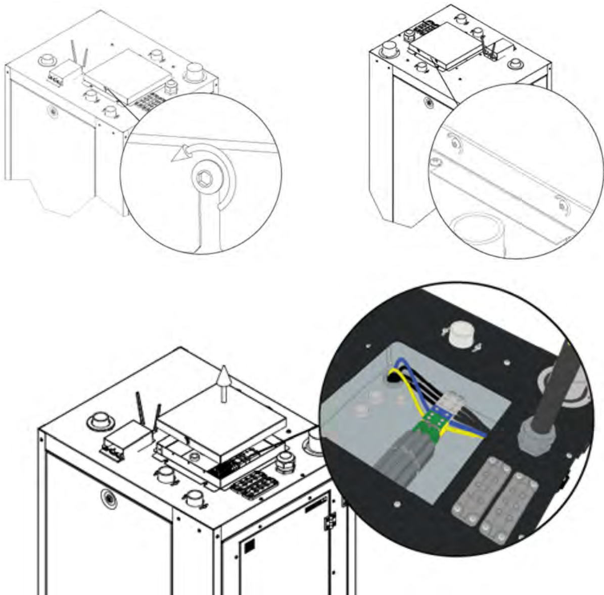
Kuva 7.3 Sähkökytkentäkotelo ja syöttökaapelin kytkentä
