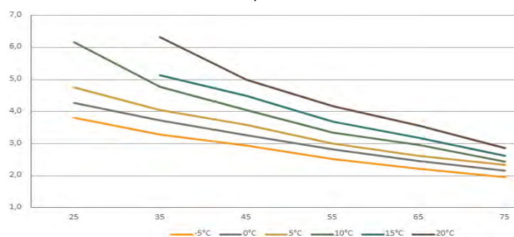
COP, 70 Hz
