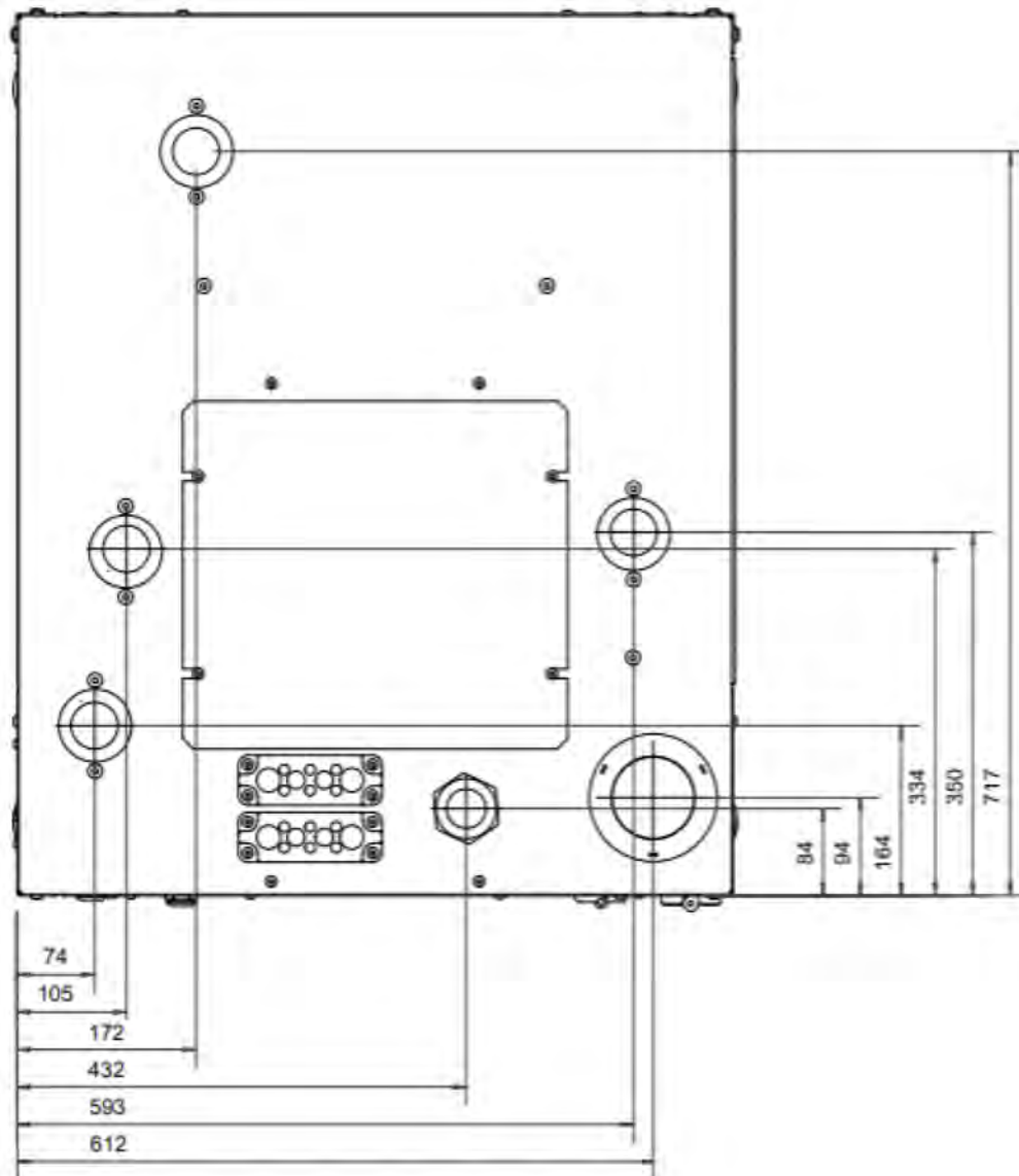
Kuva 6.3 PutkiyhTEiden asennusmitat
