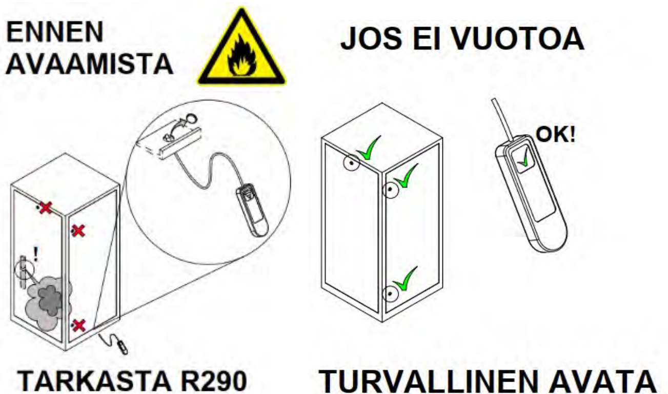
Kuva 5.12 Laitteen kylmäainevuototestaus
