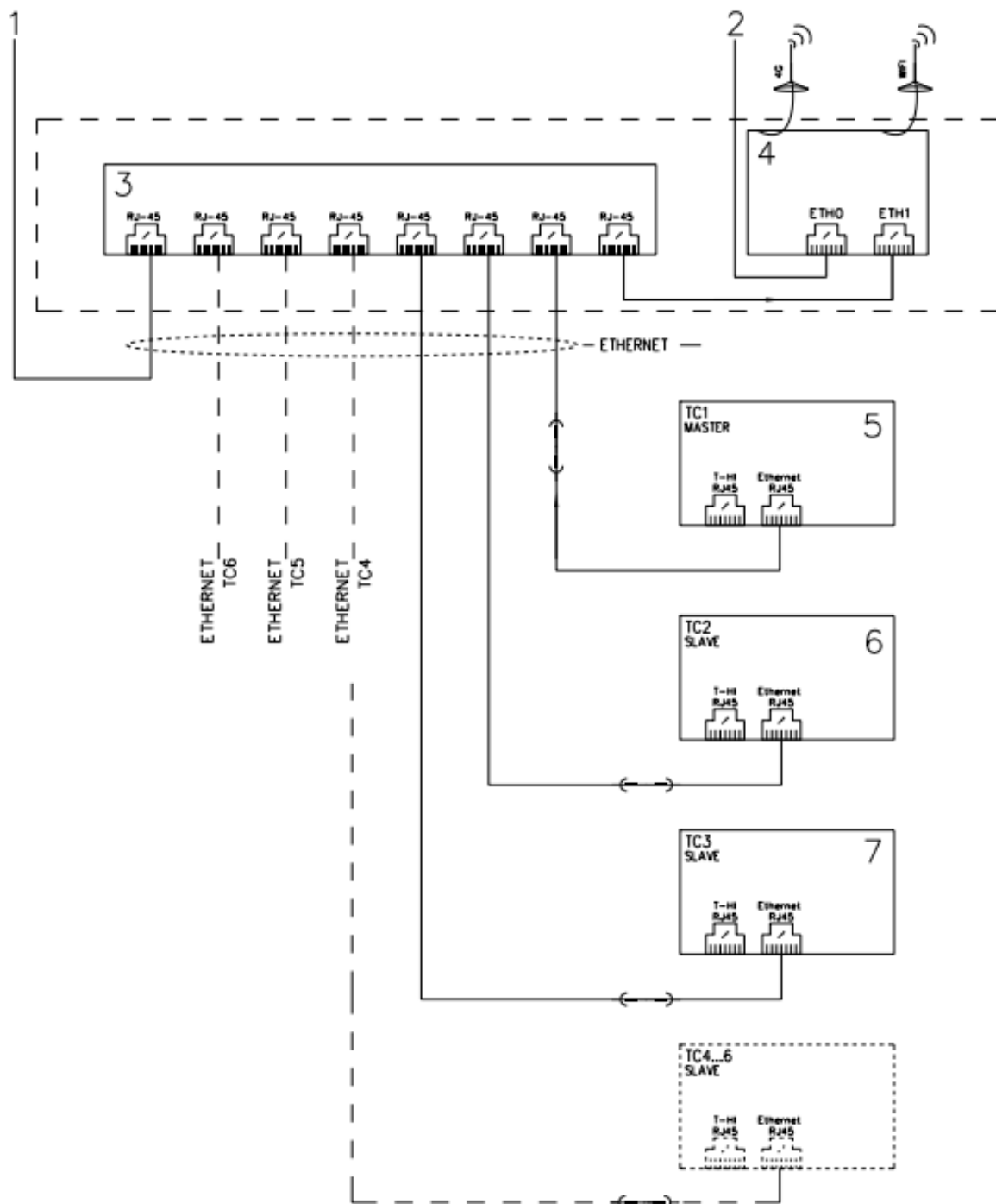
Kuva 7.4 Verkkokytinkotelo
