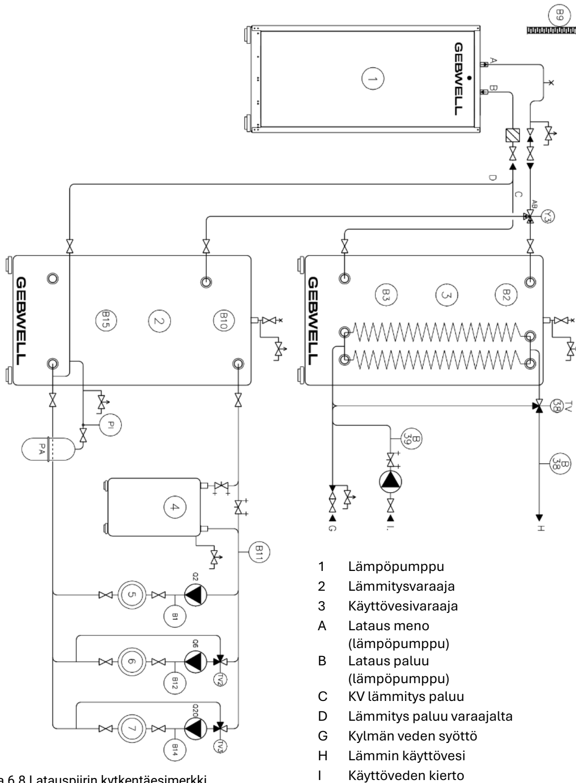
Kuva 6.8 Latauspiirin kytkentäesimerkki
