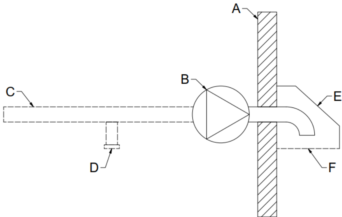
Kuva 5.11 Ilmanvaihdon ulospuhallus
