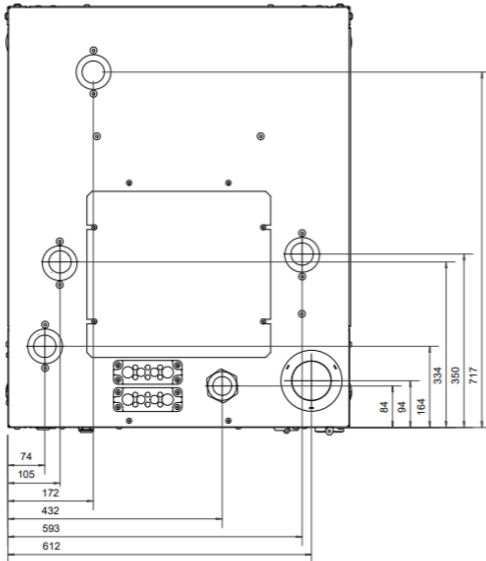
Kuva 6.3 Putkijhteiden asennusmitat
