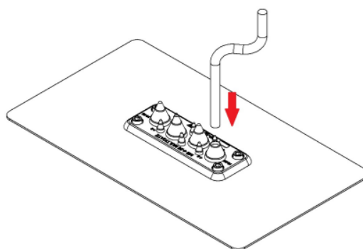
Kuva 7.2 kaapaelin asentaminen multilaippaan
