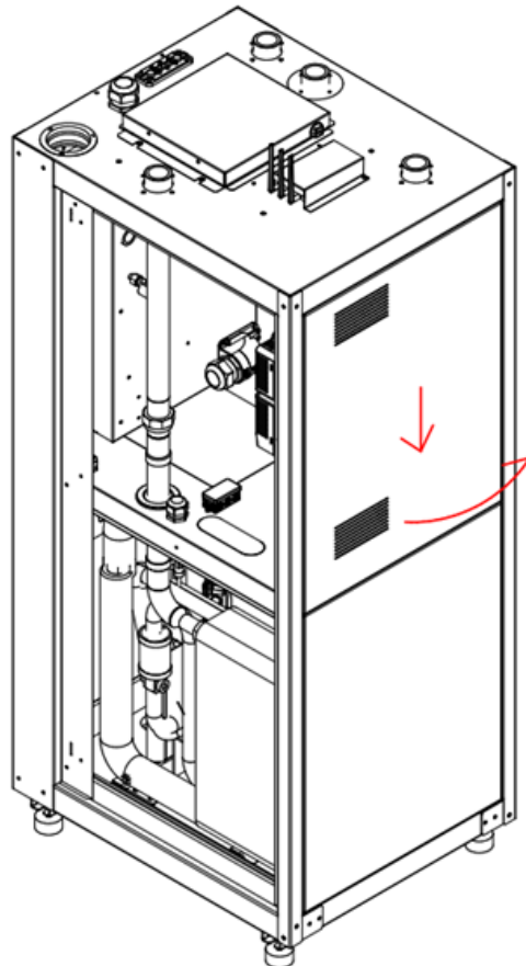
Kuva 5.18 Takaoven poistaminen
