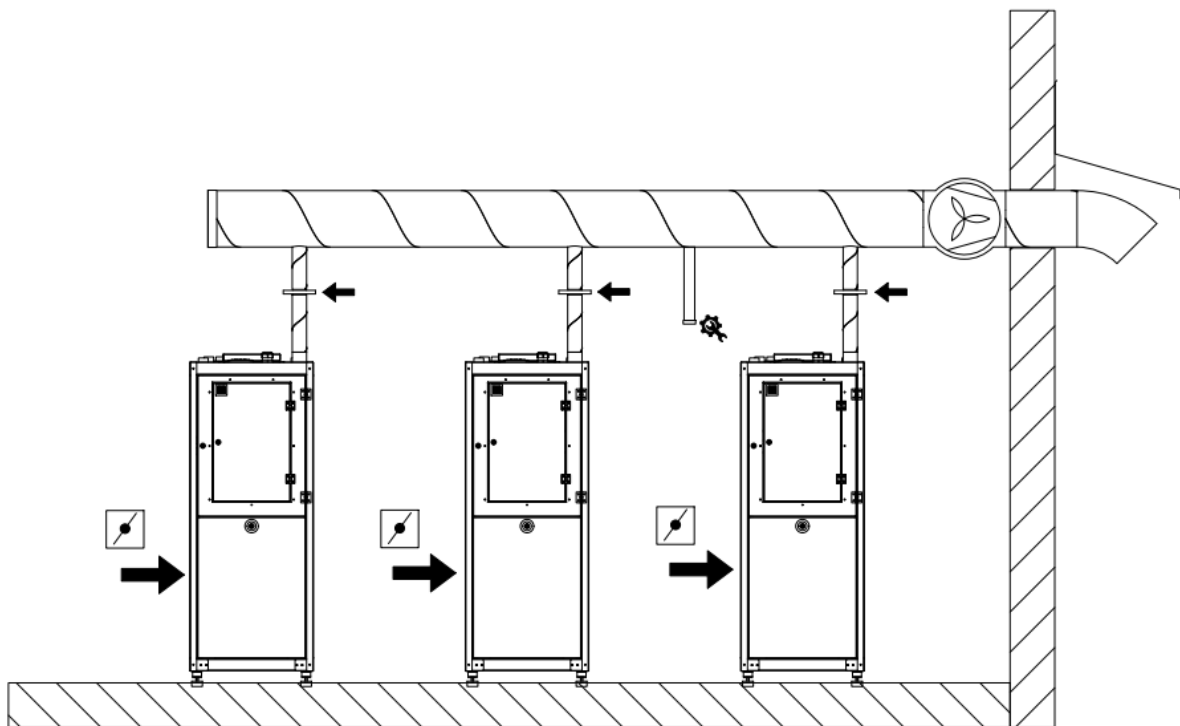
Kuva 5.10 Esimerkkikuva poistoilmaimurin ja kanavan asennuksesta kaskadijärjestelmässä
