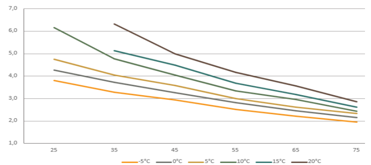
COP, 70 Hz
