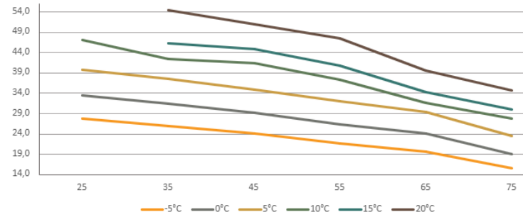
Jäähdytysteho [kW]
