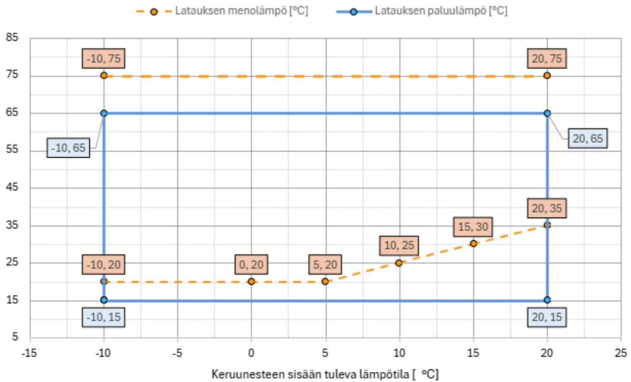
Kuva 12.1 Käyttöalue
