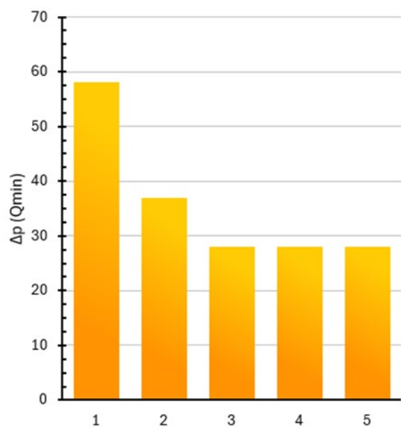
Kuvaaja 5.2 Laitteen sisäinen painehäviö ilmanvaihdolle Q_{min} virtaamalla (säätöpellin asennot 1–5)
