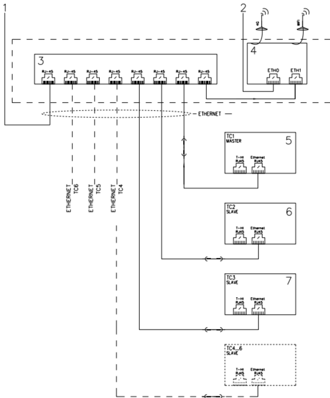
Kuva 7.4 Verkkokytkinkotelo
