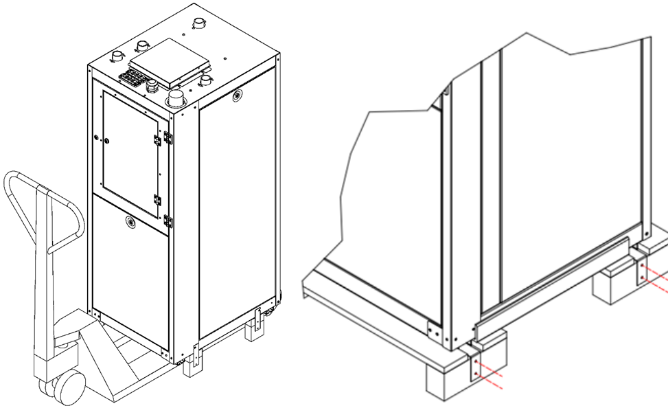
Kuva 5.4 Lämpöpumpun nostaminen ja kuljetustukien sijainti
