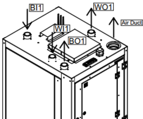
Kuva 6.1 Lämpöpumpun putkilähdöt
