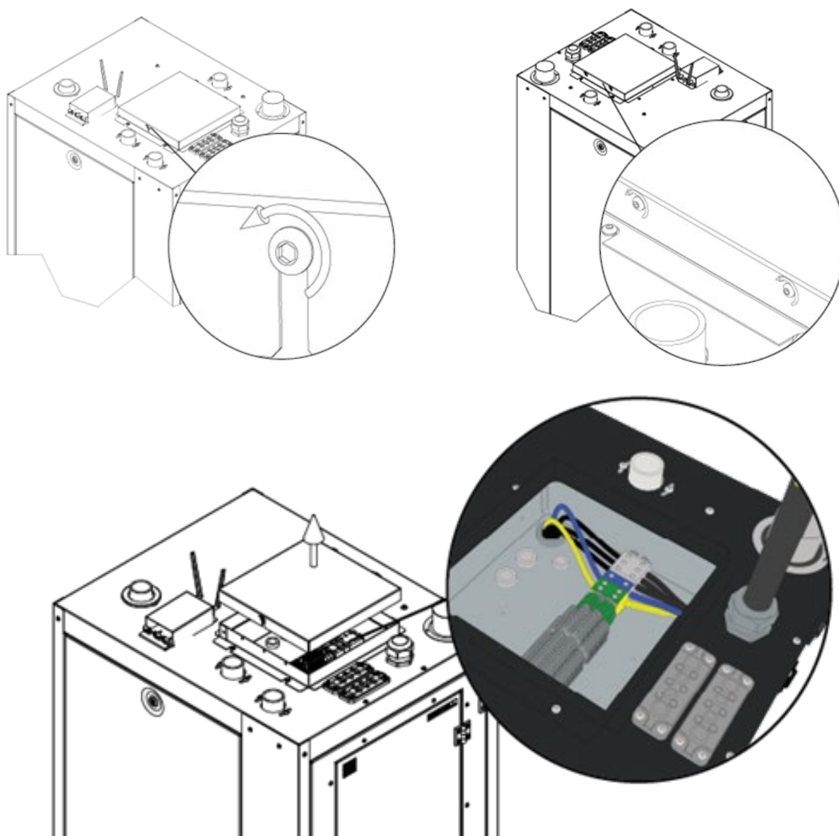
Kuva 7.3 Sähkökytkentäkotelon ja syöttökaapelin kytkentä
