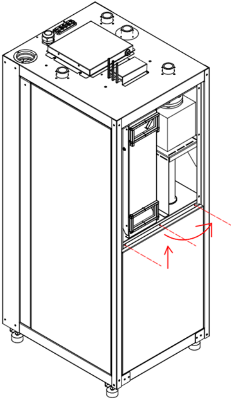
Kuva 5.19 Alemman takaoven irrottaminen
