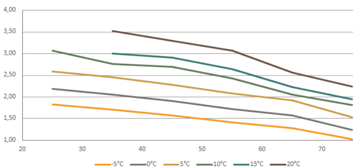
Keruupiirin virtaama dT4 [l/s]
