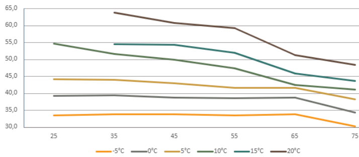
Lämmitysteho [kW]
