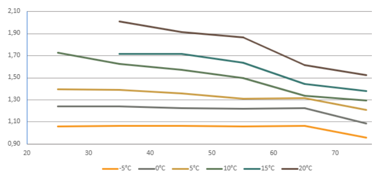
Latauspiirin virtaama dT8 [l/s]
