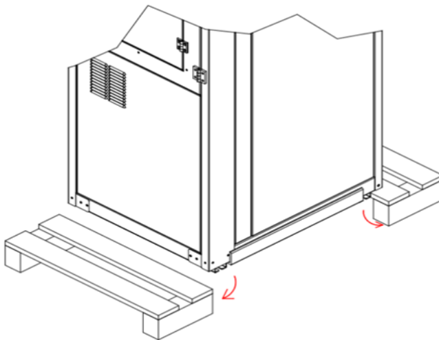
Kuva 5.5 Kuljetusalustojen poistaminen.
