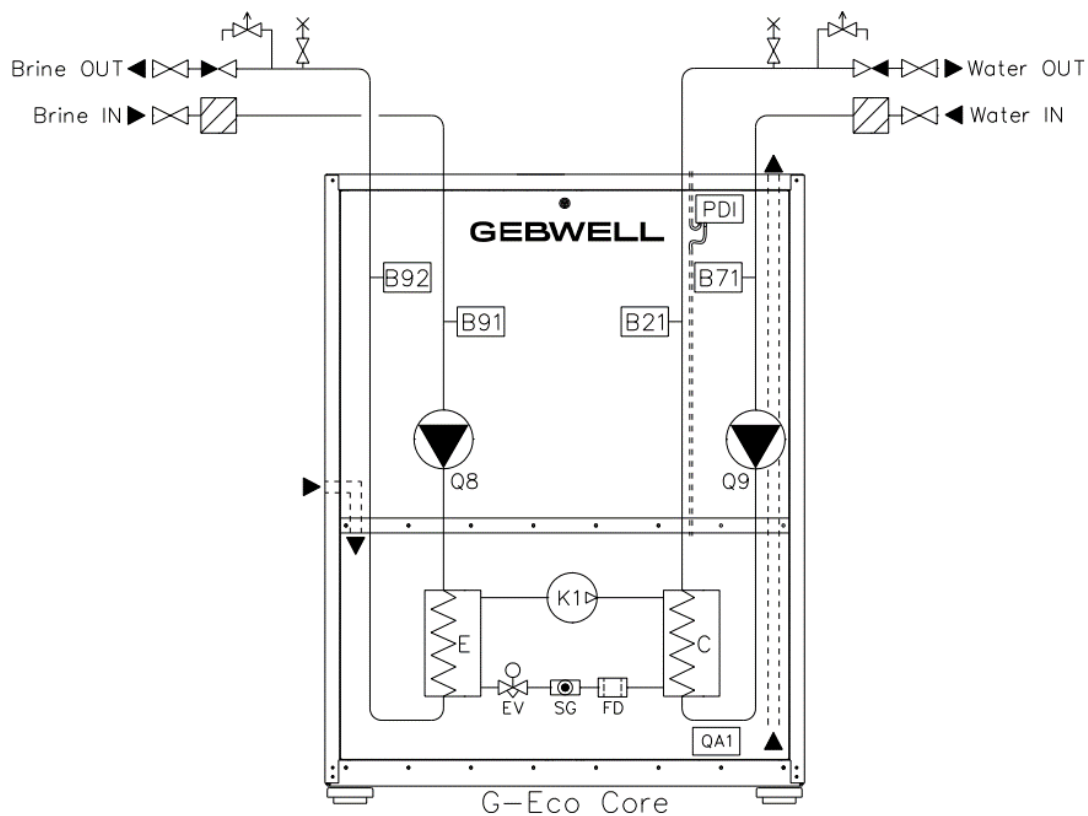
Kuva 6.2 Putkikytkentöjen mallikaavio
