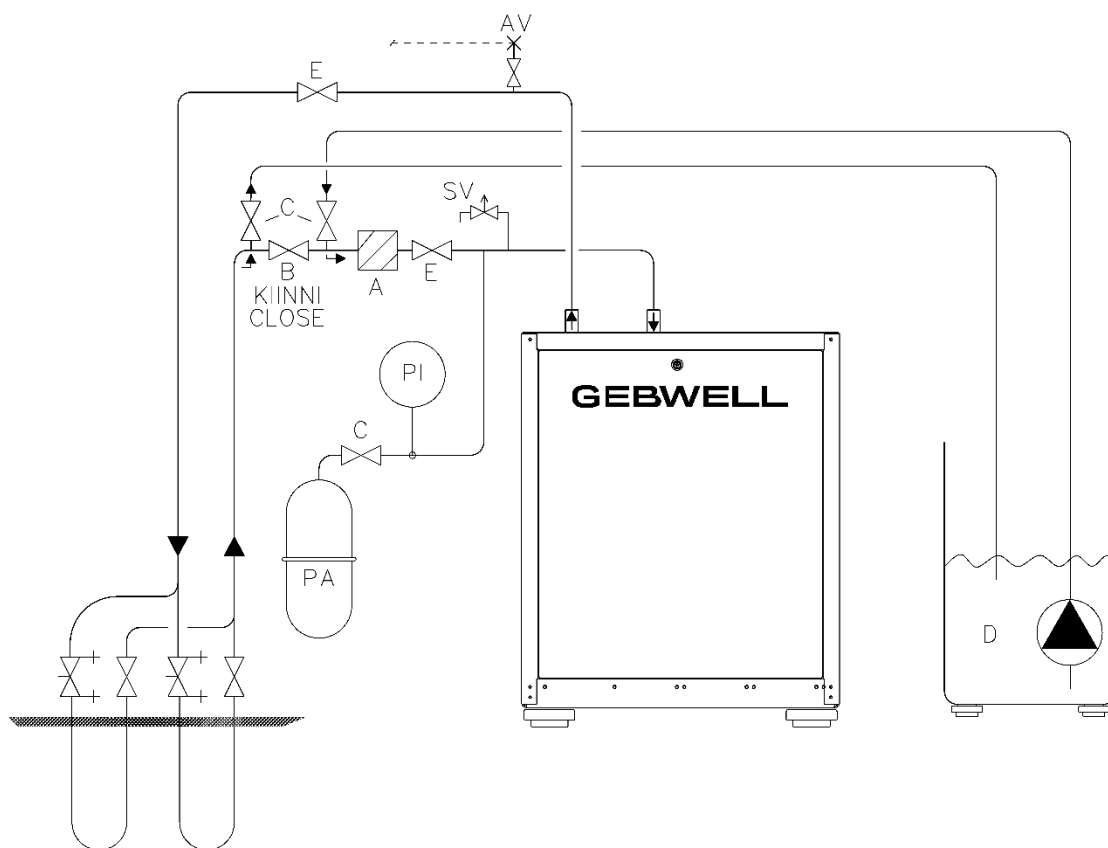
Kuva 8.1 Keruupiirin ilmaus
