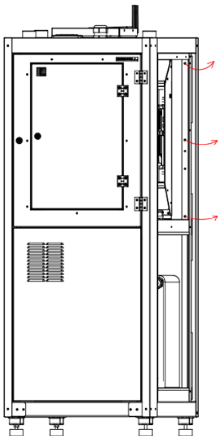
Kuva 5.17 Takaoven poistaminen
