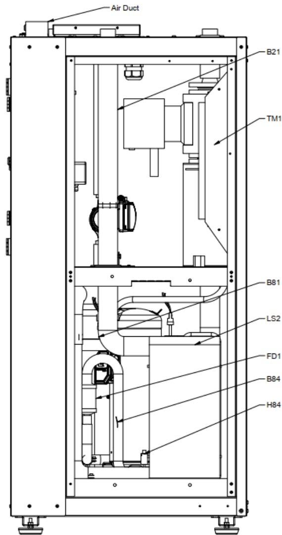
Kuva 3.5 Komponentit ja anturit (oikea)
