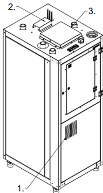
Kuva 3.3 Laitteen ulkopuoliset Komponentit ja ilmanavat
