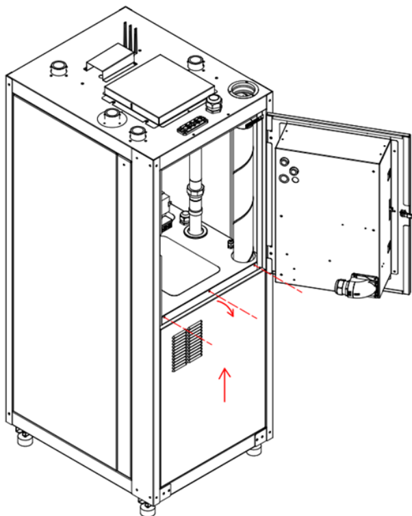
Kuva 5.16 Alemman etuoven poistaminen
