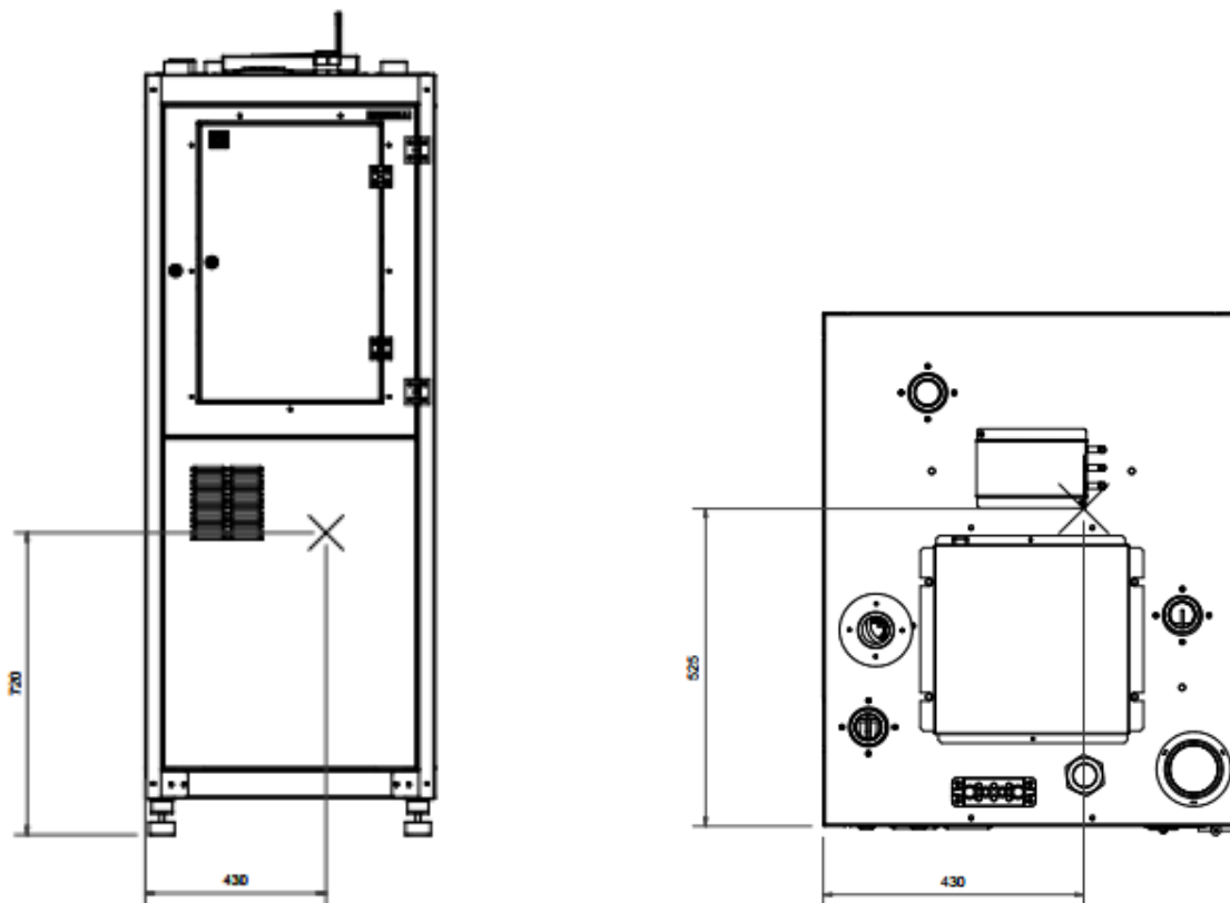
Kuva 5.1 Lämpöpumpun painopiste
