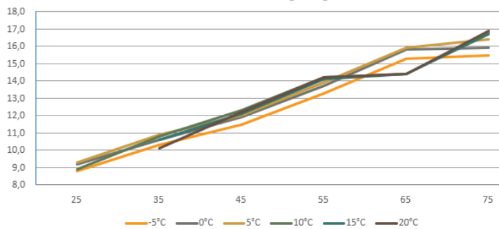
Sähköteho [kW]
