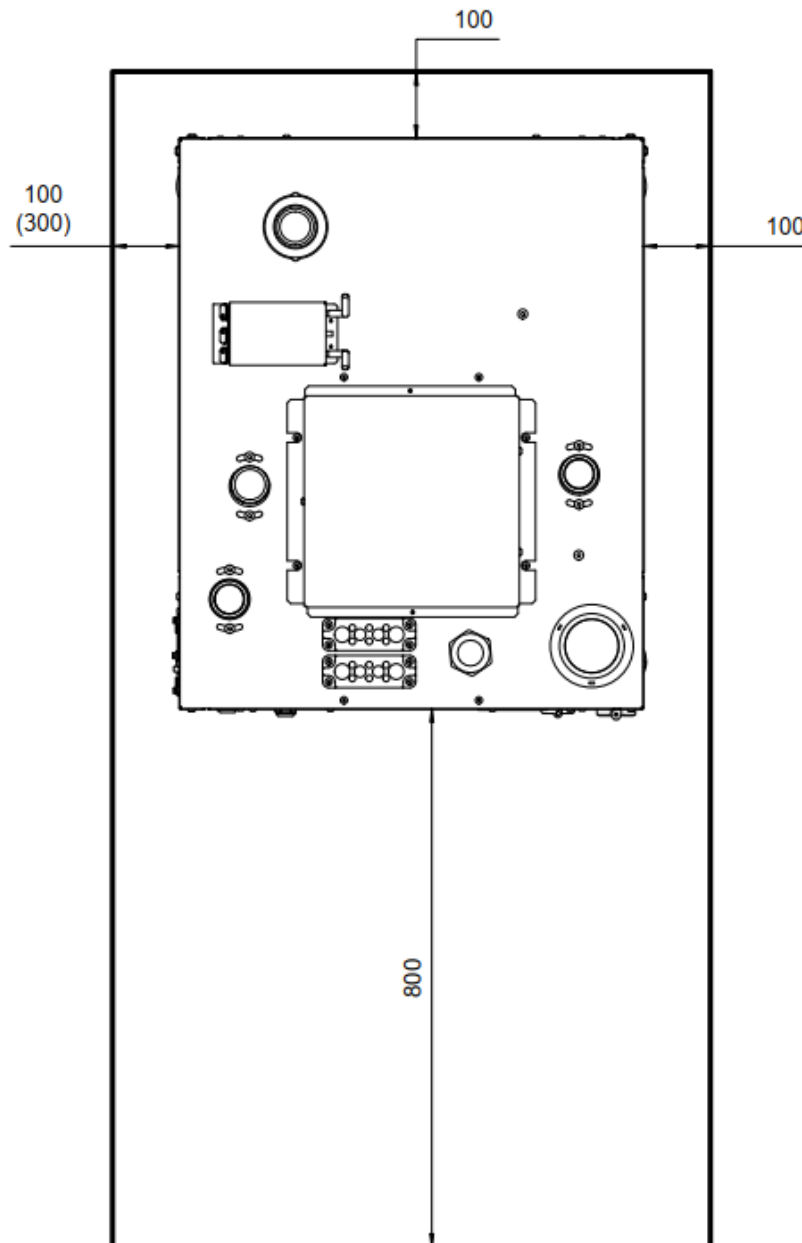
Kuva 5.6 Yhden lämpöpumpun vaatima huoltotila
