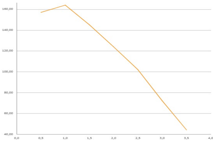
Keruupiirin virtaama dT4 [l/s]
