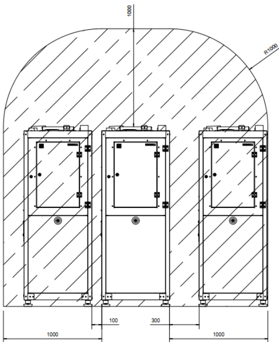
Kuva 5.9 Tilaluokiteltu alue kylmäpiiriin kohdistuvan huollon yhteydessä (useampi lämpöpumppu)
