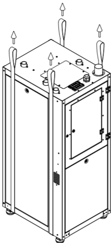
Kuva 5.2 Liinanosto
