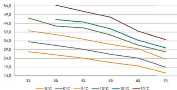
COP, 70 Hz
