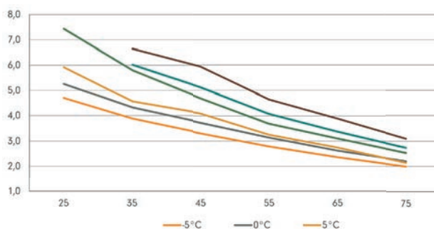
COP, 70 Hz
