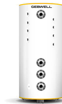
G-Energy Buffertank SV 1000 L 8SV DN65
