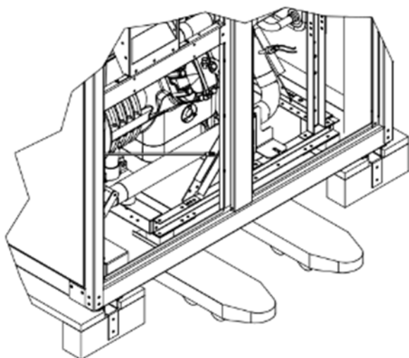
Bild 5.6 Avlägsna transportunderlagen
