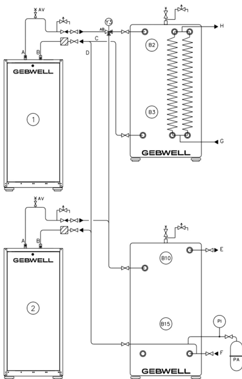
Bild 6.7 Exempelbild, kaskadanslutning
