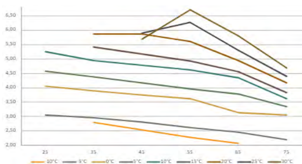
Flöde i laddkretsen dT8 [l/s]
