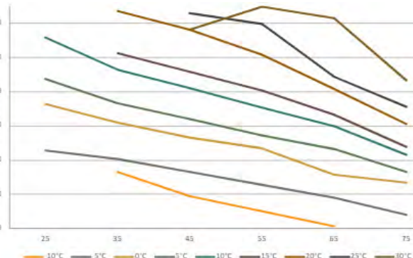
Kyleffekt [kW]
