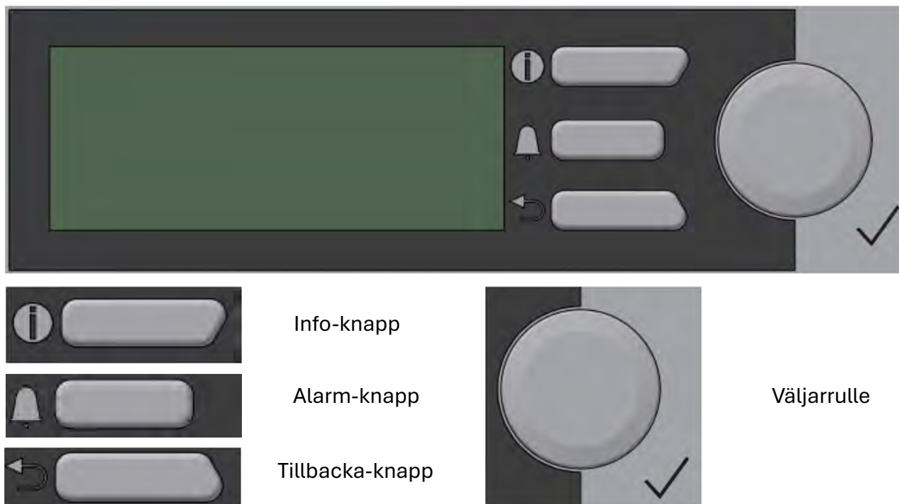
Bild 9.1 Reglerenhetens användargränssnitt
