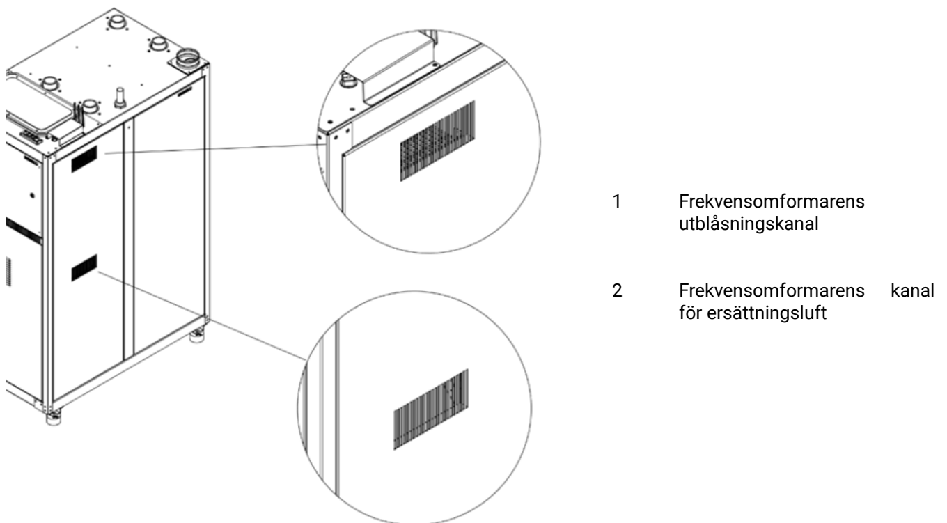
Bild 3.3 Frekvensomformarens ventilationskanaler
