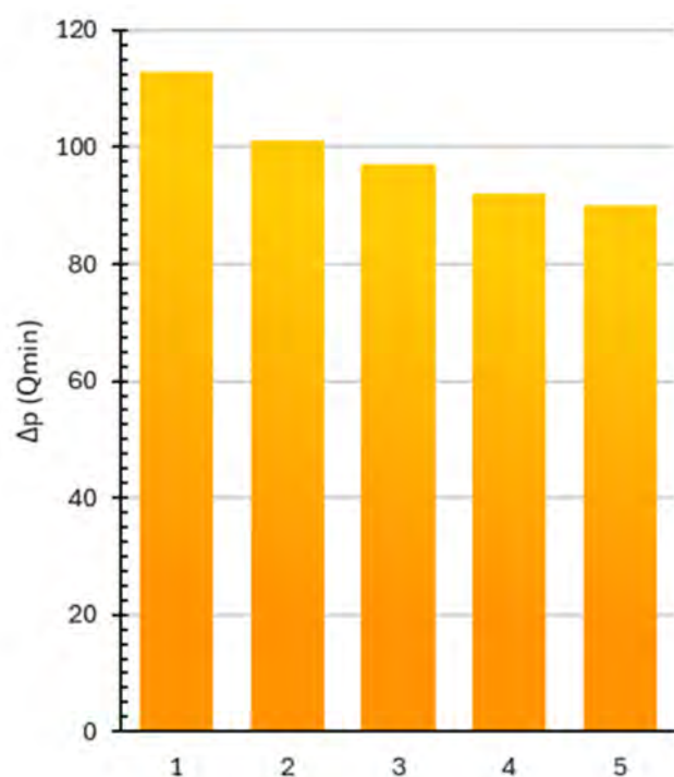
Diagram 5.2 Intern tryckförlust för ventilation vid Qmin (164 m³/h) flöde (spjällinställningar 1-5)
