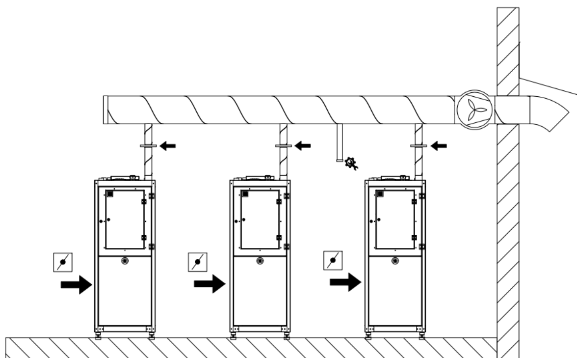
Bild 5.14 Exempelbild på installation av frånluftsfäkt och kanal i kaskadsystem
