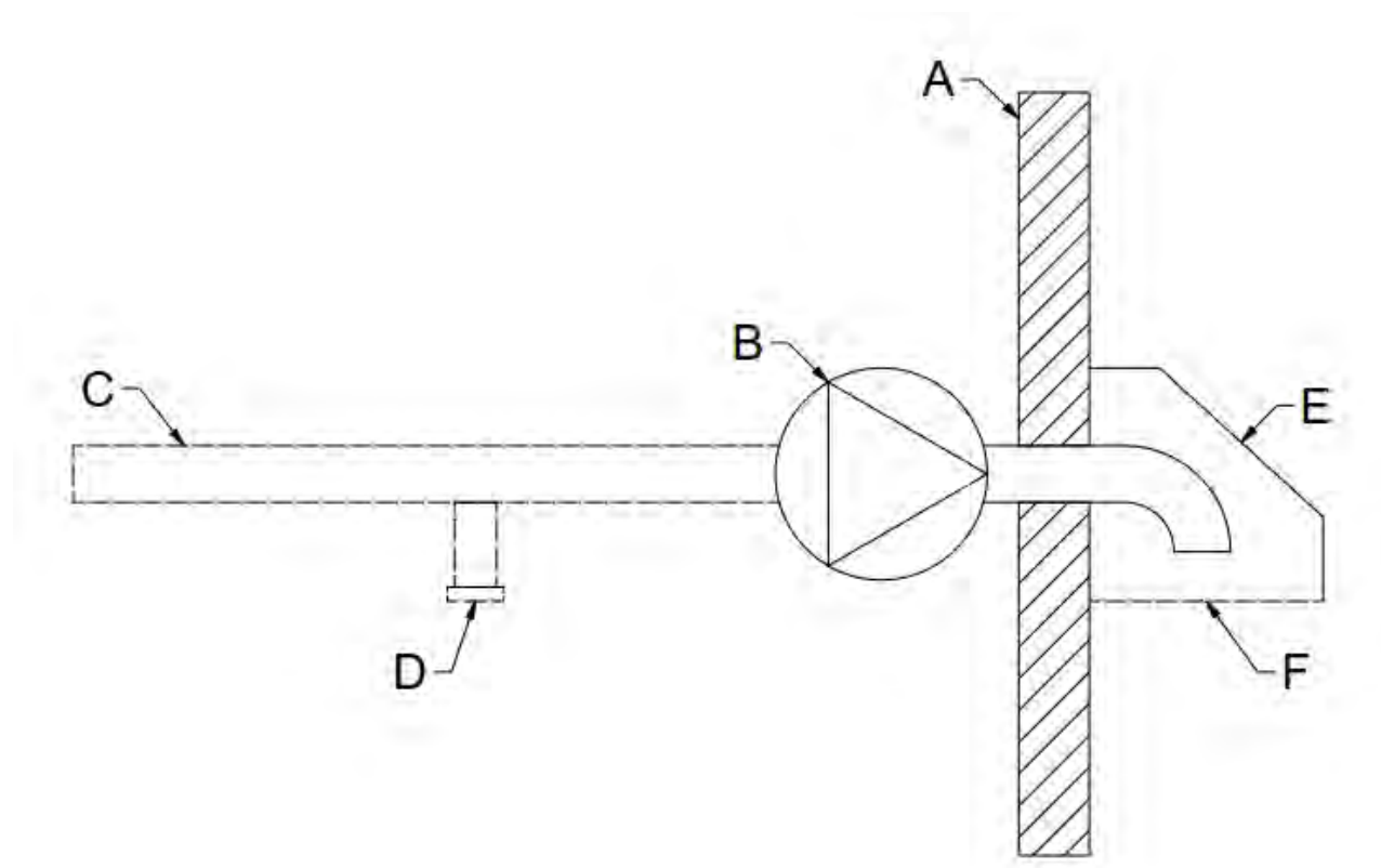
Bild 5.15 Utblås från ventilationen
