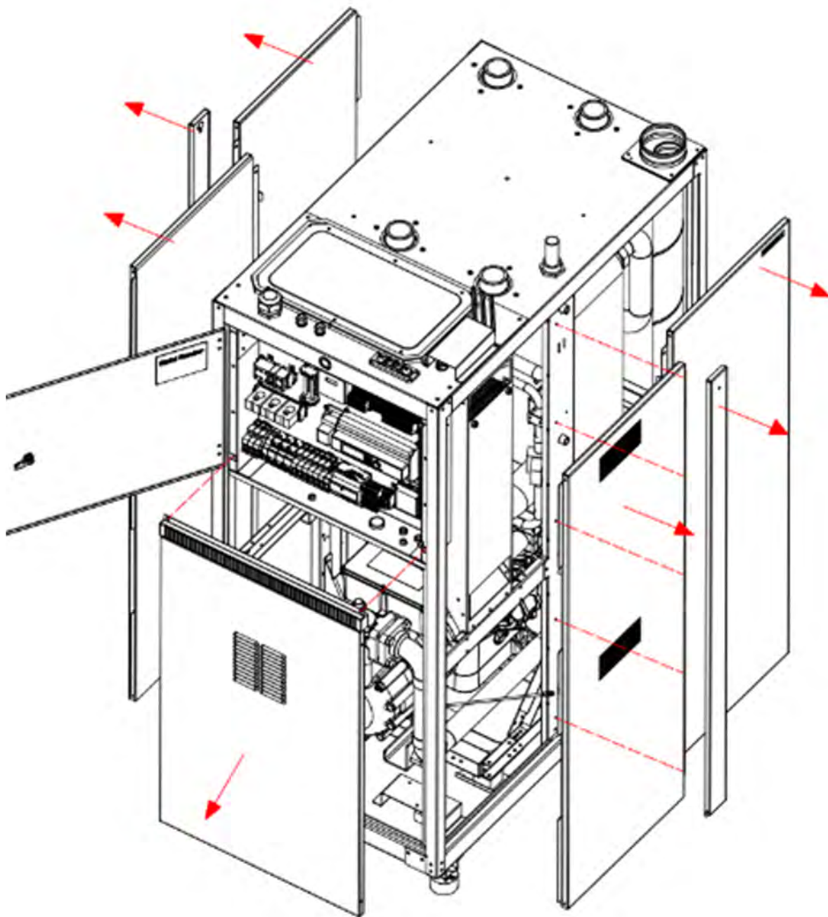
Bild 5.17 Demontering av höljesplåtar
