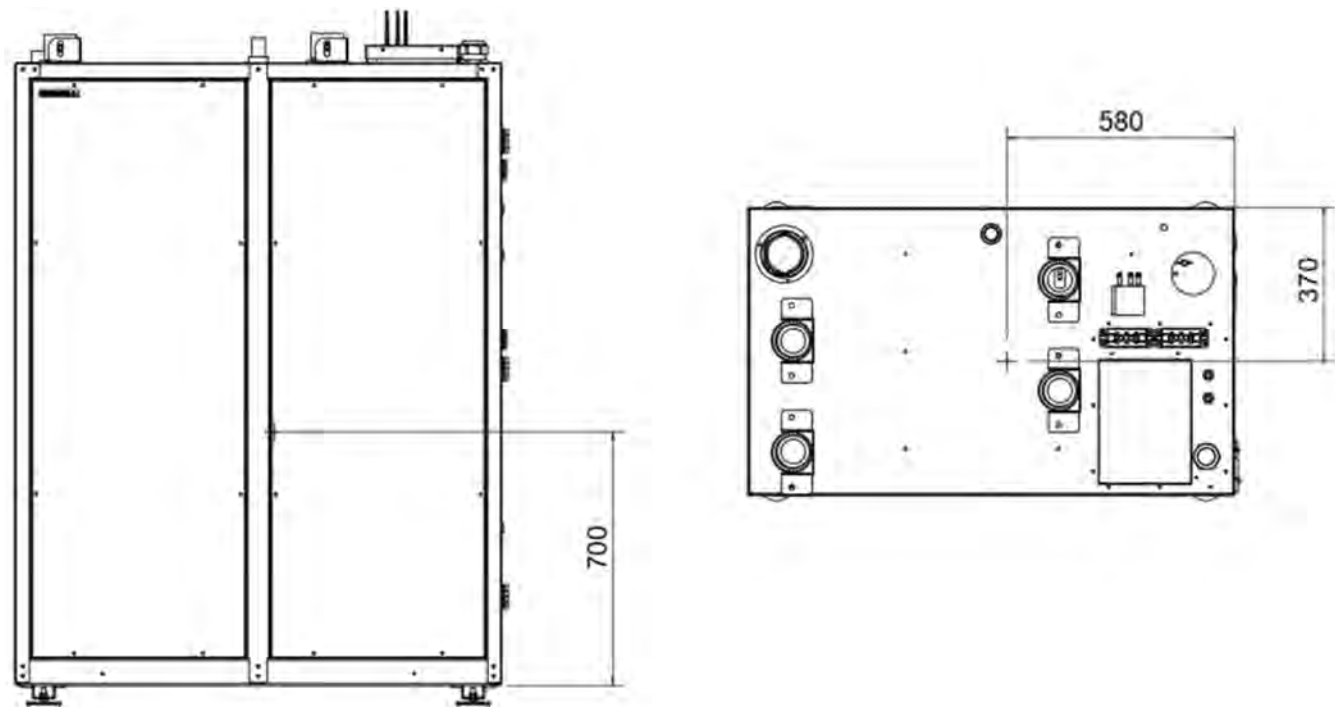
Bild 5.1 Värmepumpens tyngdpunkt
