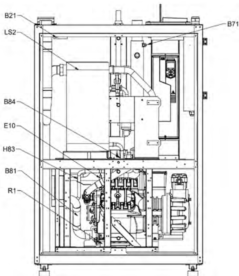
Bild 3.4 Komponenter och givare (vänster)
