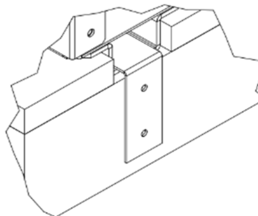
Bild 5.5 Transportstödens placering
