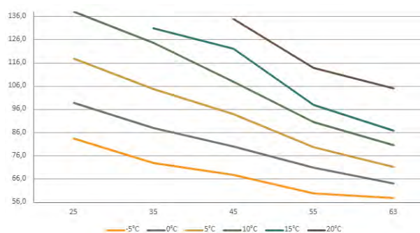
COP, 70 Hz
