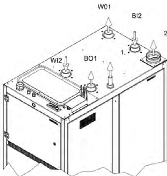
Bild 6.1 Värmepumps rörutgångar
