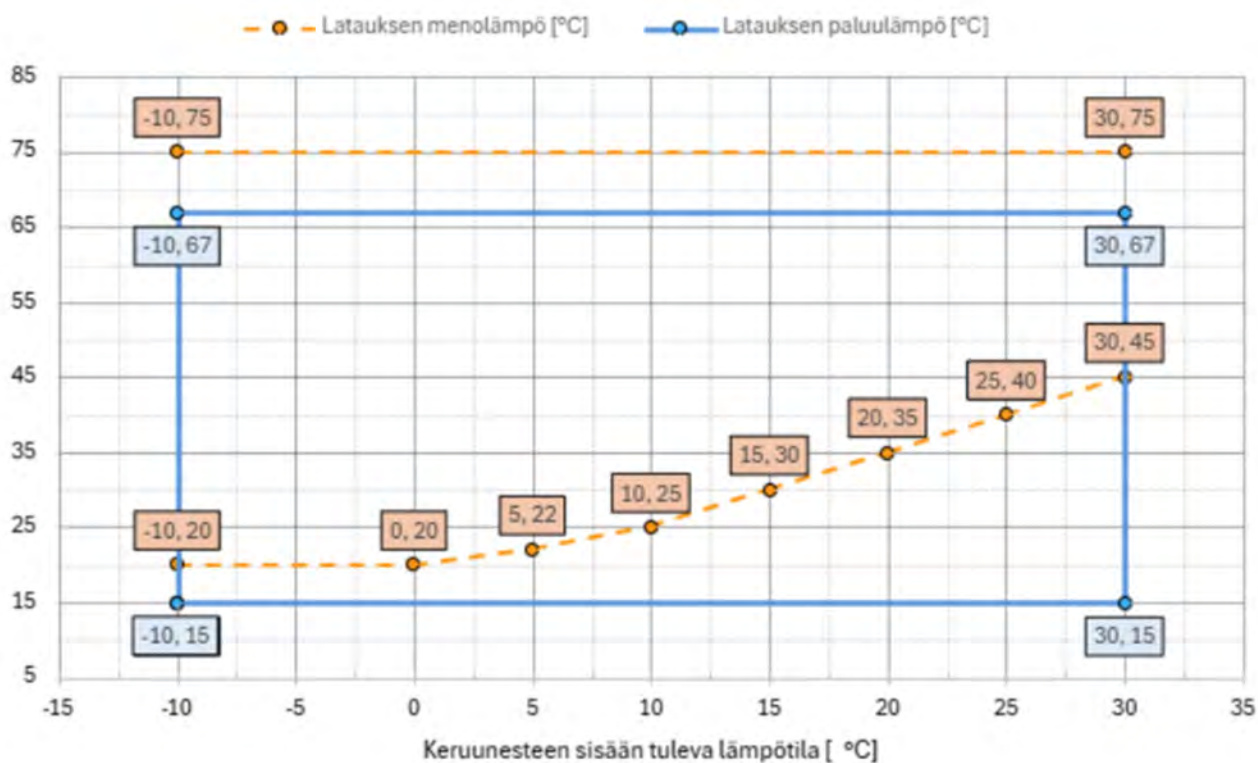
Bild 12.2 Driftområde G-Eco Pro 120 HT
