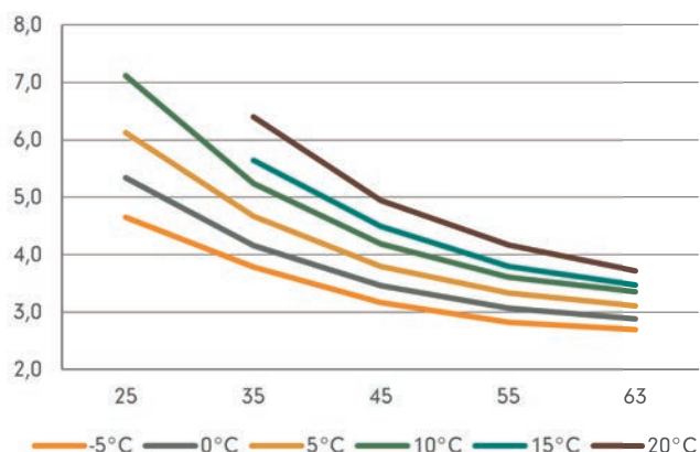
COP, 50 Hz
