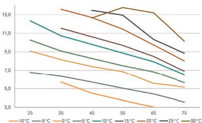
Kollektor flöde dT3 [l/s]
