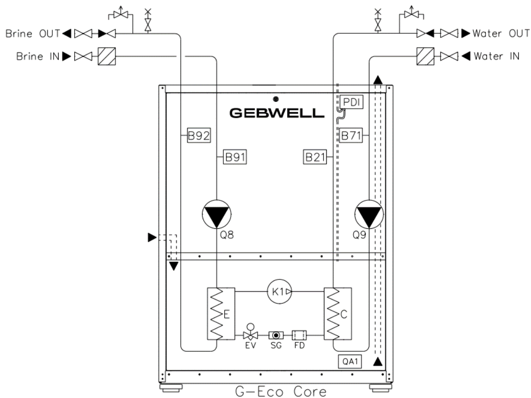
Kuva 6.2 Putkikytentöjen mallikaavio
