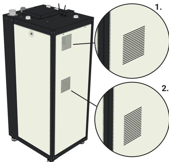
Kuva 3.3 Taajuusmuuttajan ilmanvaihtokanavat
