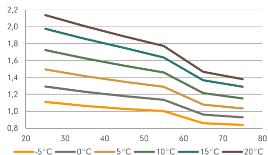
Latauspiirin virtaama dT8 [l/s]
