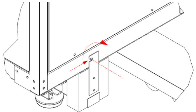
Kuva 5.4 Lämpöpumpun nostaminen ja kuljetustukien sijainti
