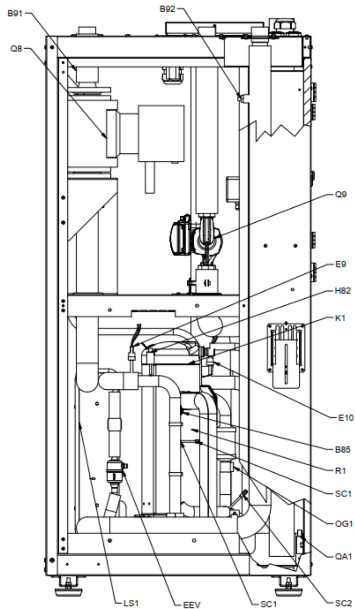
Kuva 3.4 Komponentit ja anturit (vasen)
