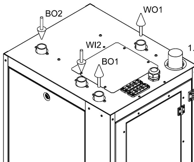
Kuva 6.1 Lämpöpumpun putkilähdöt
