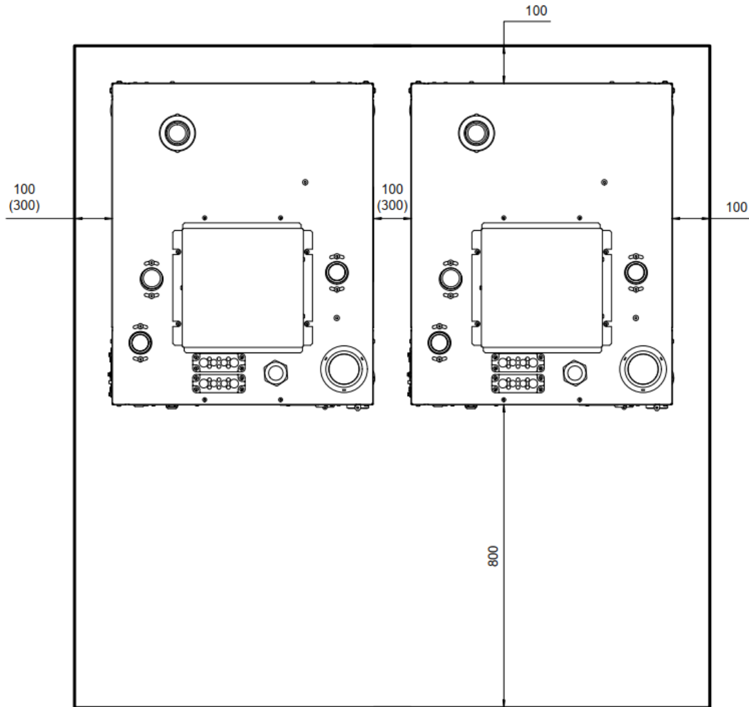
Kuva 5.8 Kahden lämpöpumpun vaatima huoltotila
