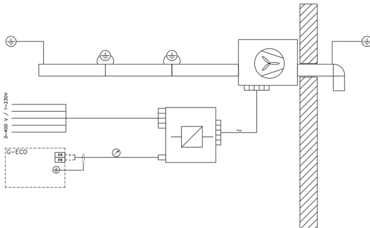
Kuva 7.5 Poistoilmamurin kytkentäkaavio
