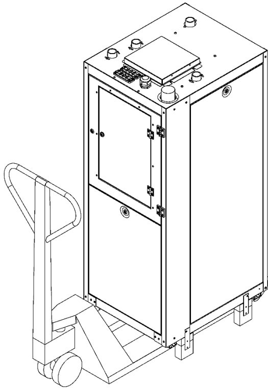
Kuva 5.4 Lämpöpumpun nostaminen ja kuljetustukien sijainti
