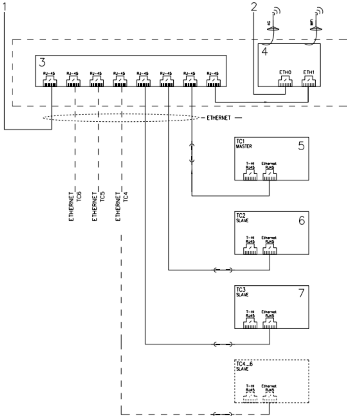
Kuva 7.4 Verkkokytinkotelo
