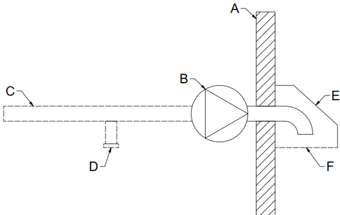
Kuva 5.12 Ilmanvaihdon ulospuhallus
