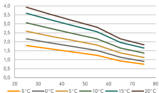
Keruupiirin virtaama dT4 [l/s]
