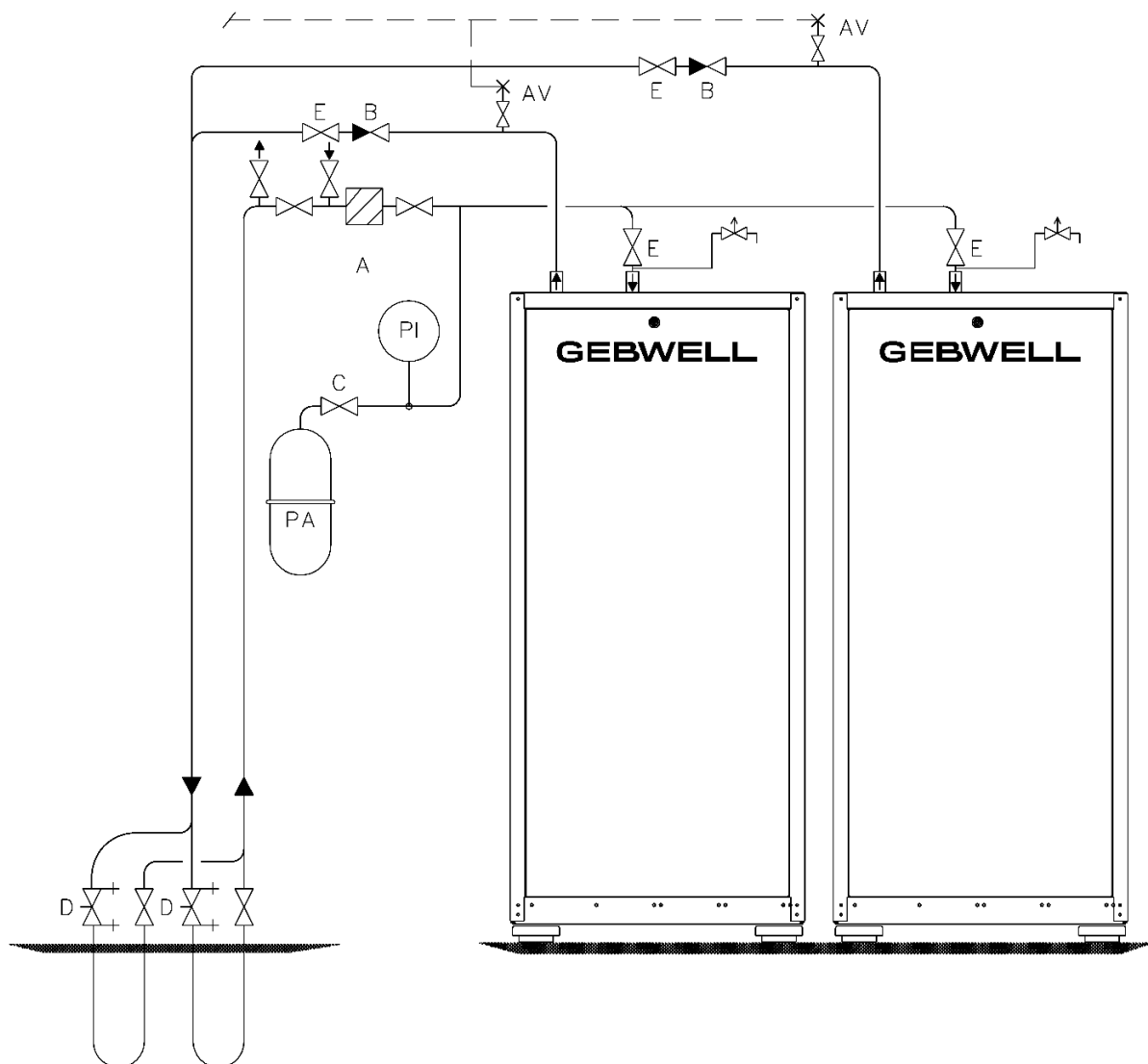
Kuva 6.6 Keruupiirin kytettä, kaksi laitetta
