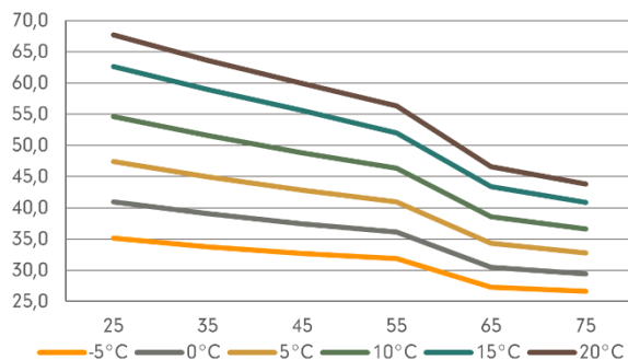
Sähköteho [kW]
