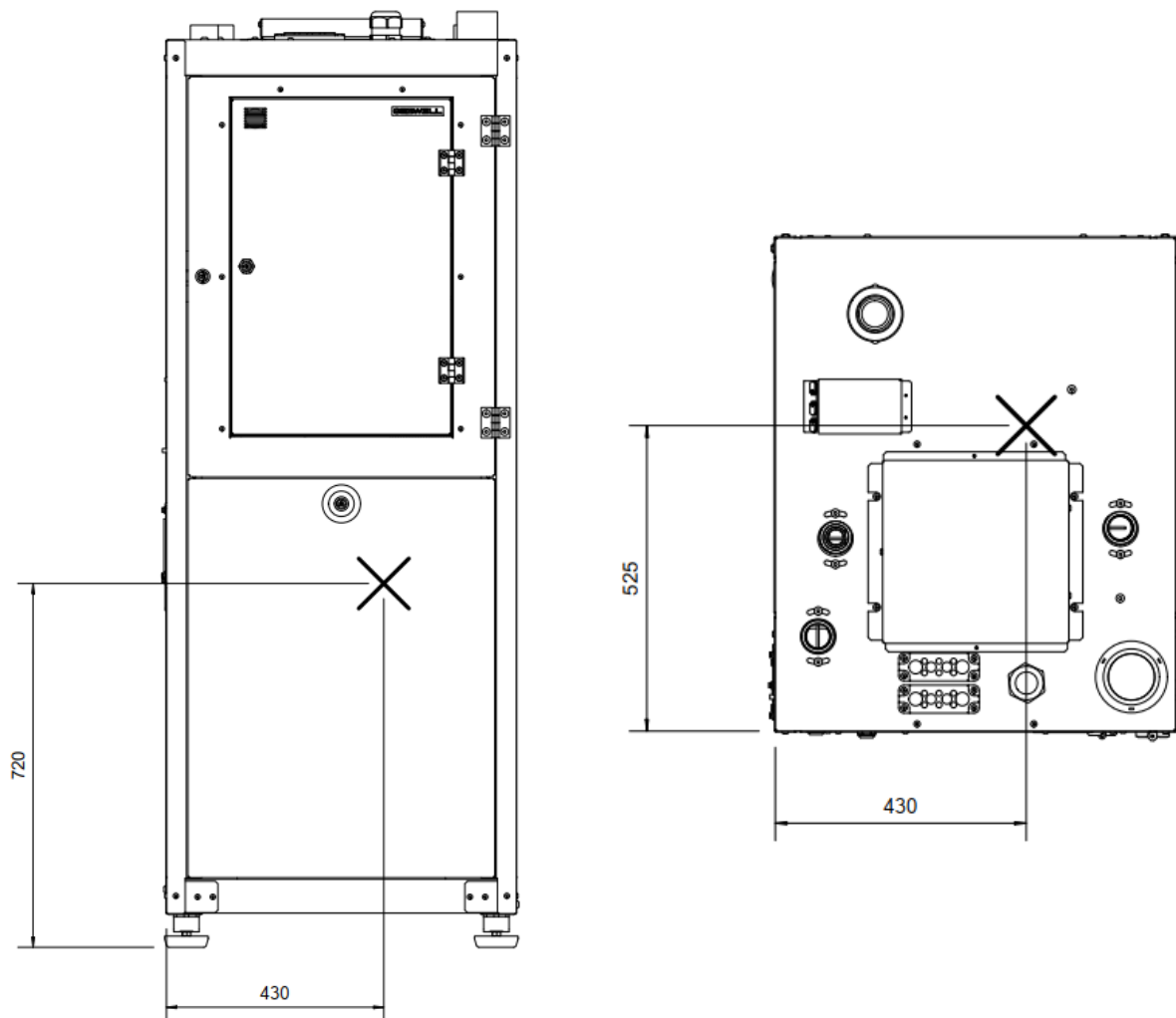
Kuva 5.1 Lämpöpumpun painopiste
