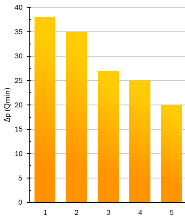
Kuvaaja 5.2 Laitteen sisäinen painehäviö ilmanvaihdon Q_{min} virtaamalla (säätöpellin asennot 1–5)
