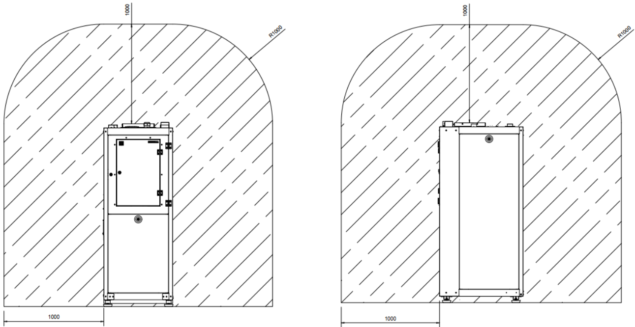
Kuva 5.9 Tilaluokiteltu alue kylmäpiiriin kohdistuvan huollon yhteydessä (edestä ja sivusta)
