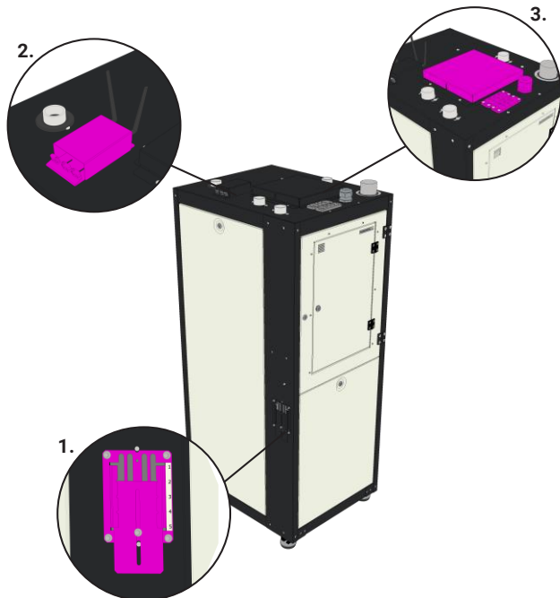
Kuva 3.2 Laitteen ulkopuoliset Komponentit ja ilmakeinavat
