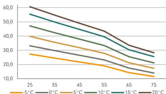
COP, 70 Hz
