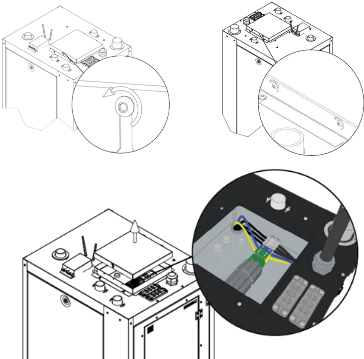
Kuva 7.3 Sähkökytkentäkotelon ja syöttökaapelin kytkentä
