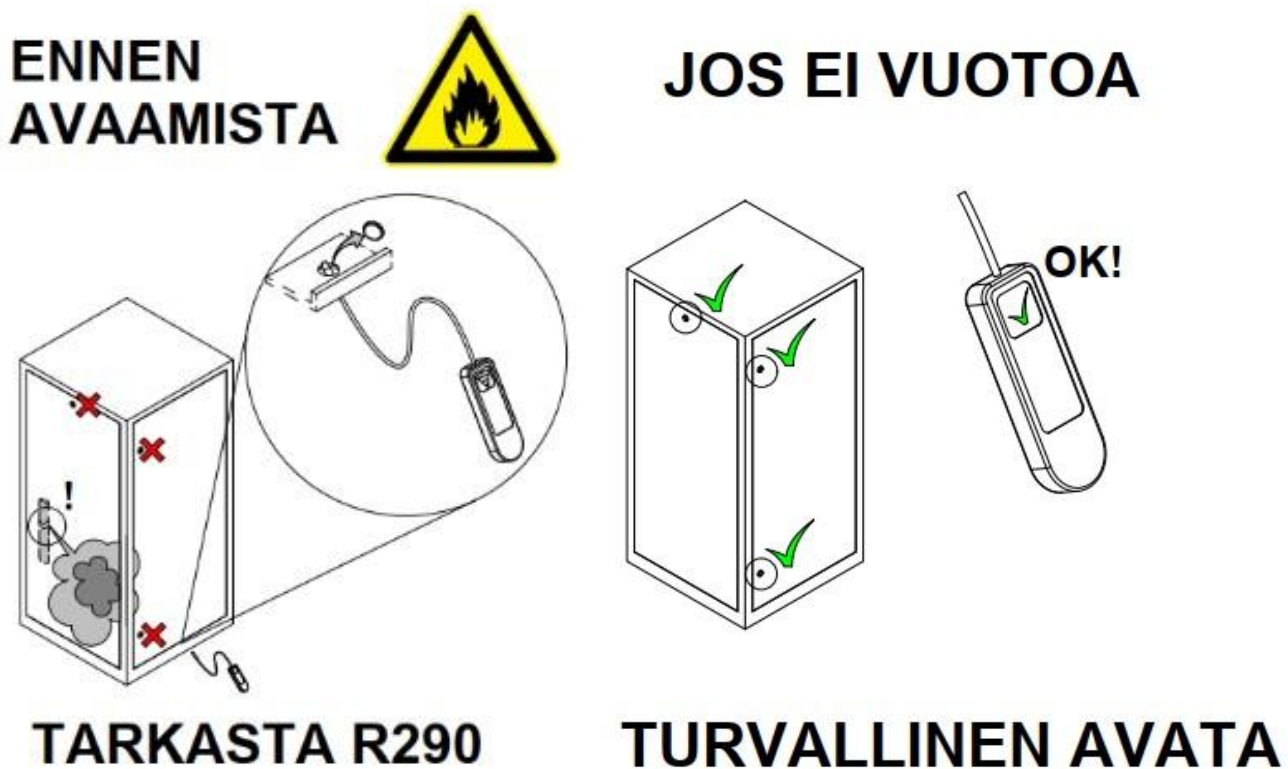
Kuva 5.13 Laitteen kylmäainevuototestaus
